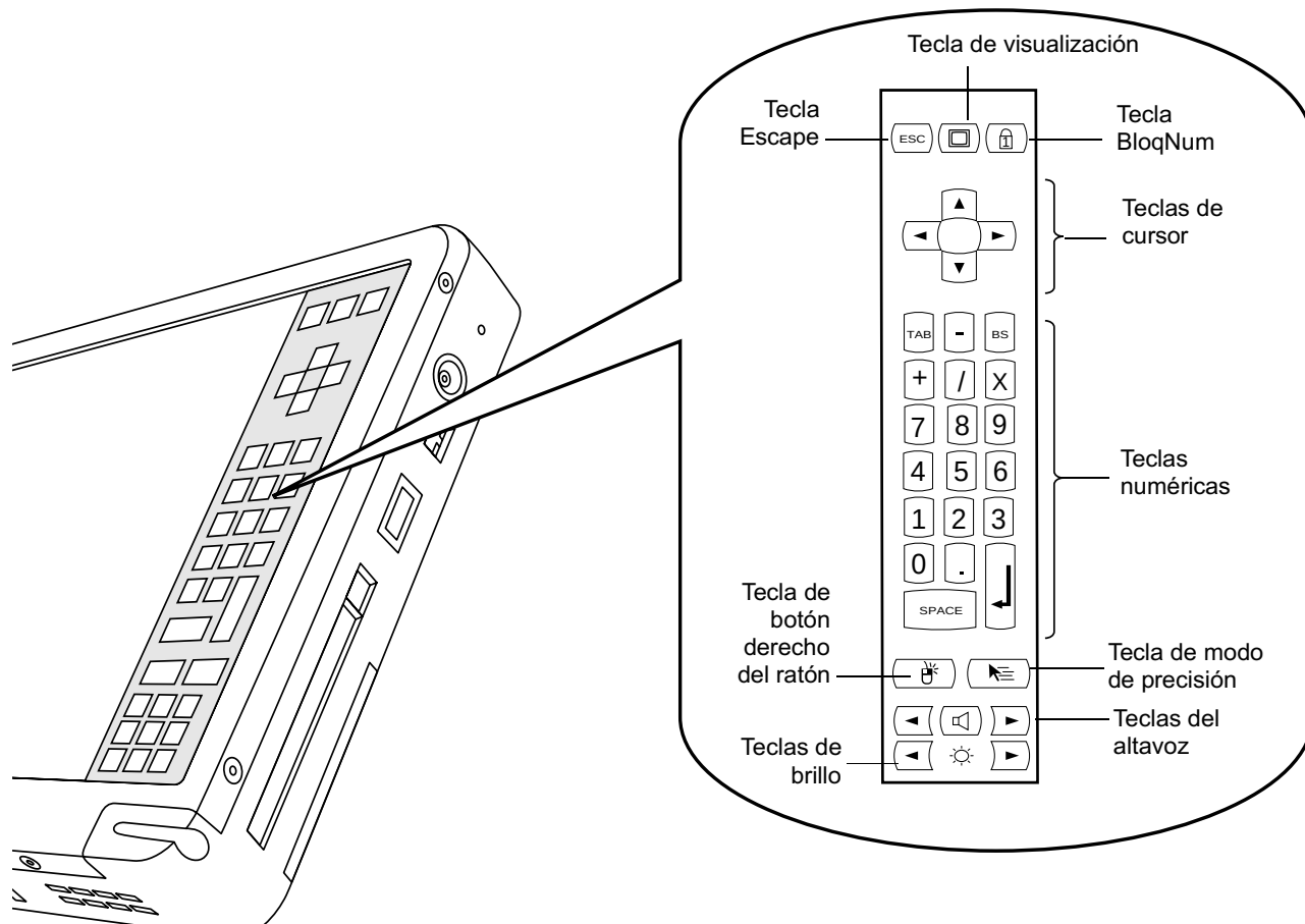
Figura 2-1 Hotpads del Stylistic
