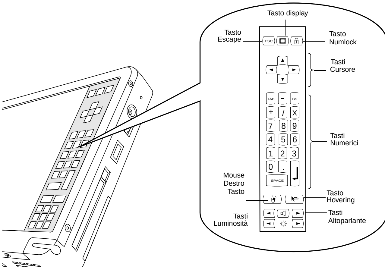
Figura 2-1 Serie tasti di regolazione di StylisticLT C-500
