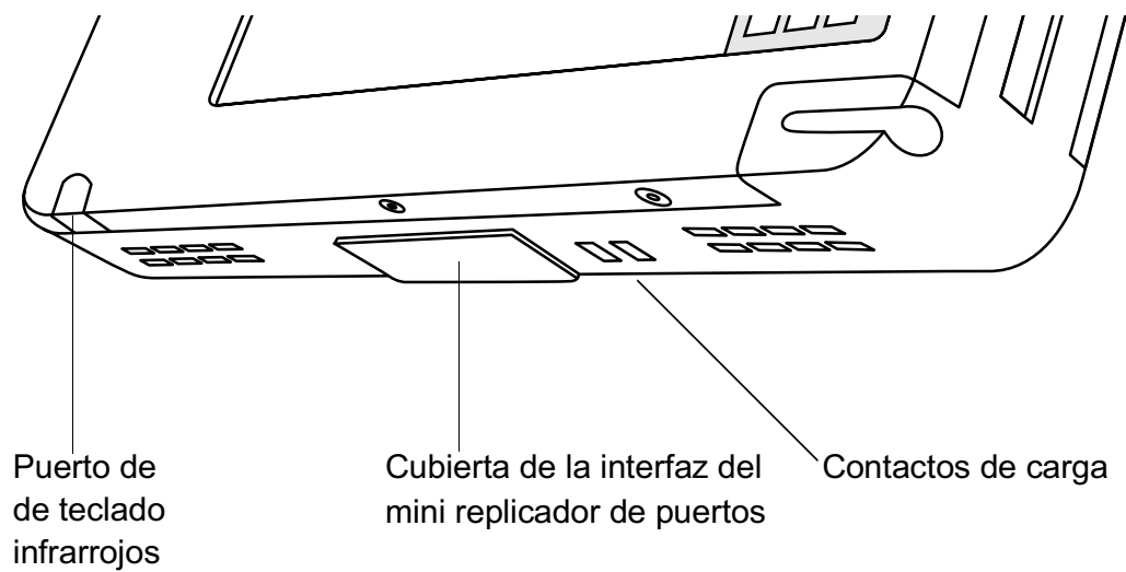
Figura 1-6 Conectores e interfaces de la parte inferior
