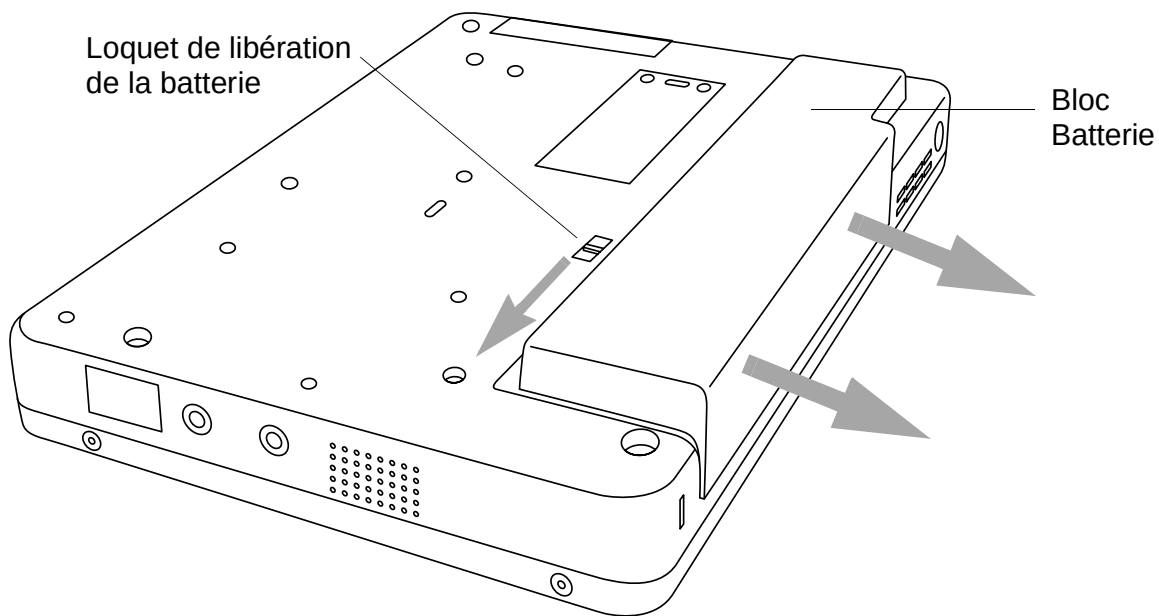
Figure 2-2 Extraction du bloc batterie
