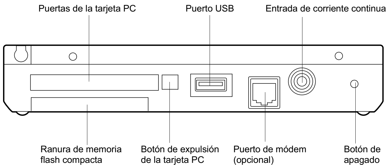
Figura 1-4 Conectores e interfaces del lateral derecho
