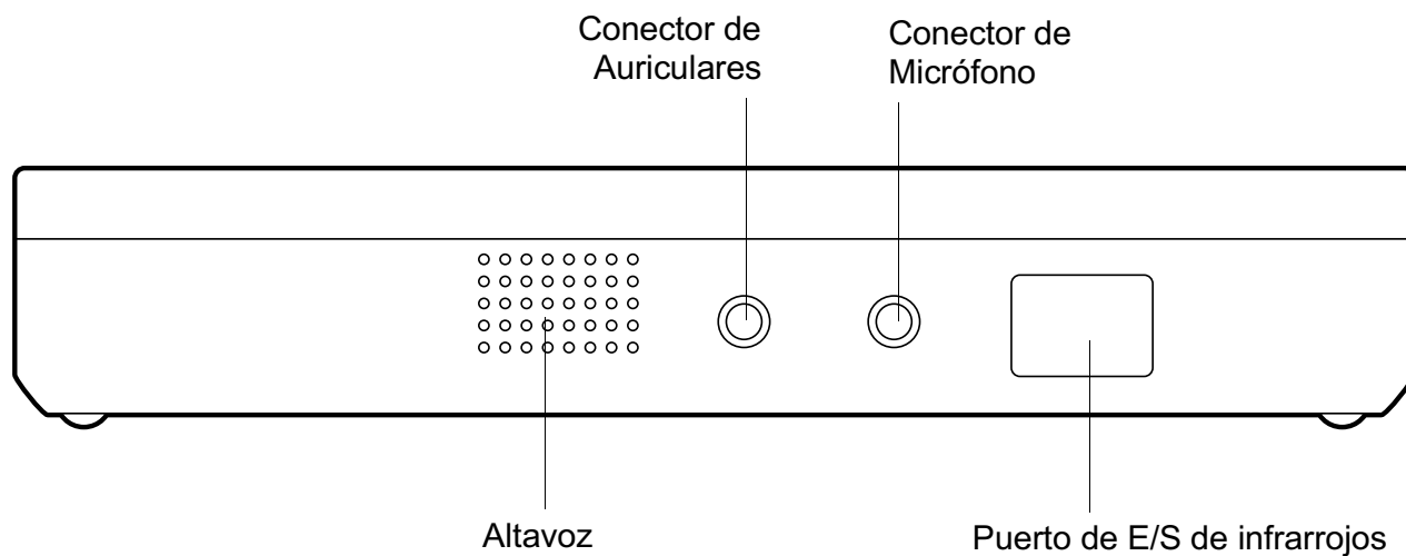
Figura 1-5 Conectores e interfaces del lateral izquierdo
