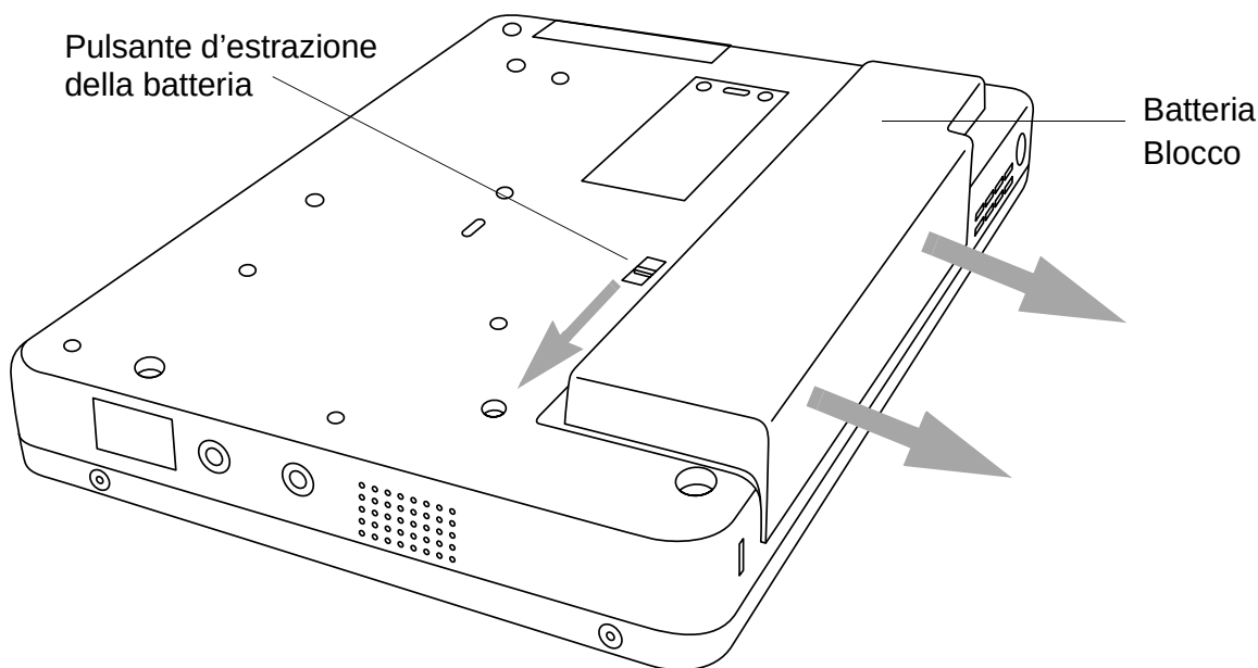
Figura 2-2 Rimozione del blocco batterie
