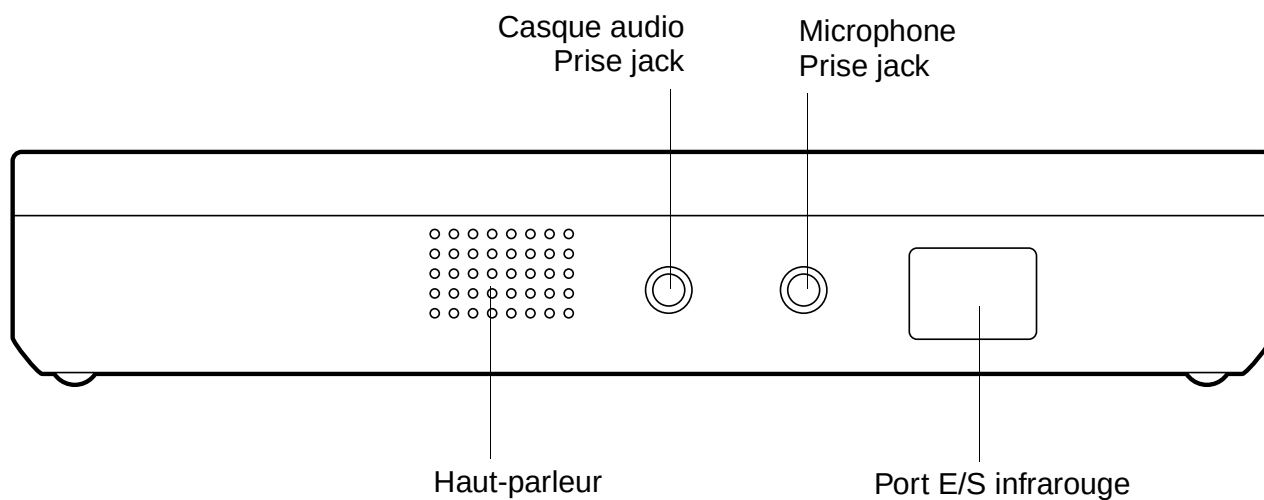
Figure 1-5 Connecteurs et interfaces du côté gauche
