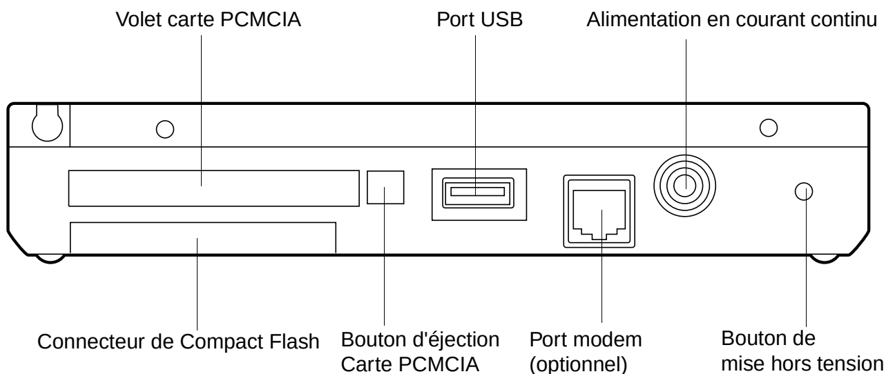
Figure 1-4 Connecteurs et interfaces du côté droit
