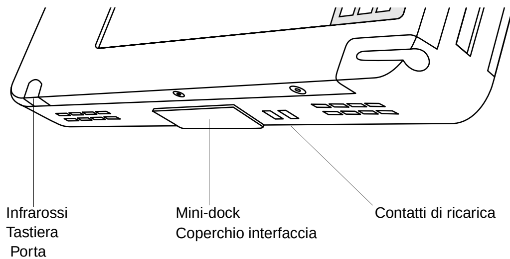
Figura 1-6 Connettori e interfacce sul fondo
