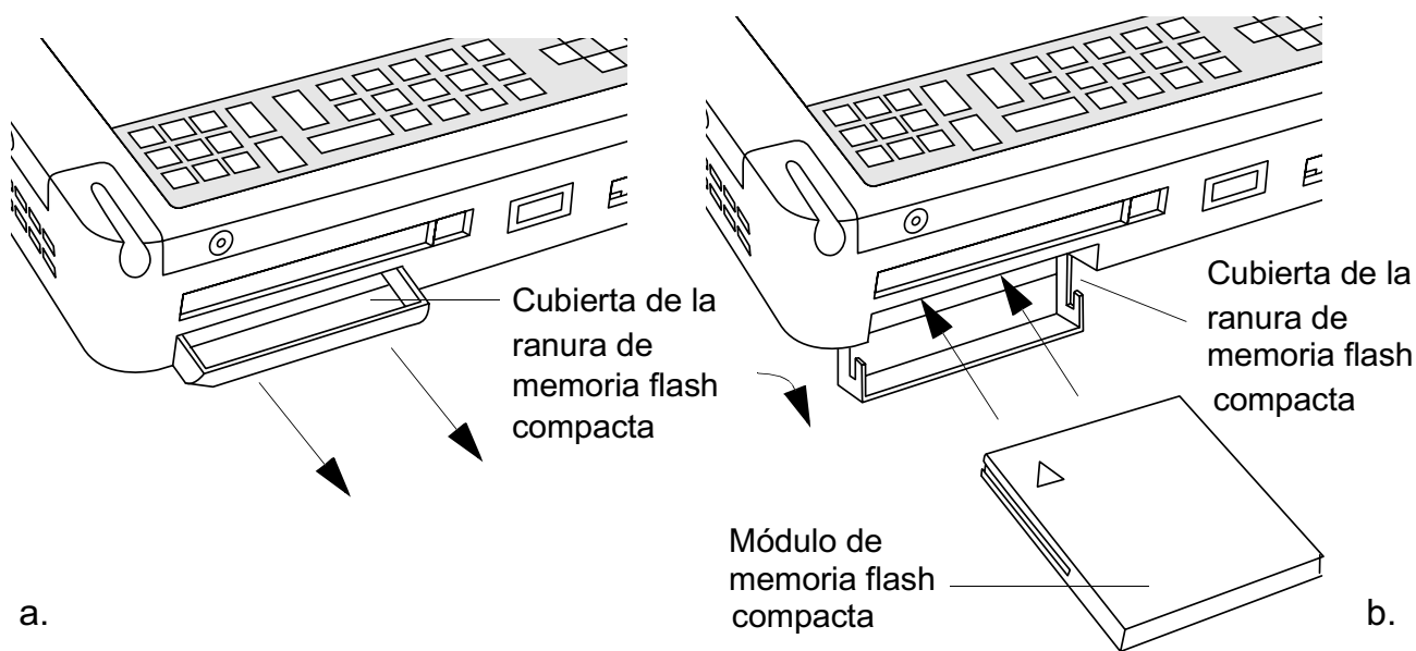
Figura 2-3 Instalación del módulo de memoria flash compacta
