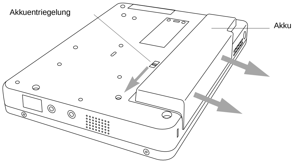
Abbildung 2-2 Entfernen des Akkus
