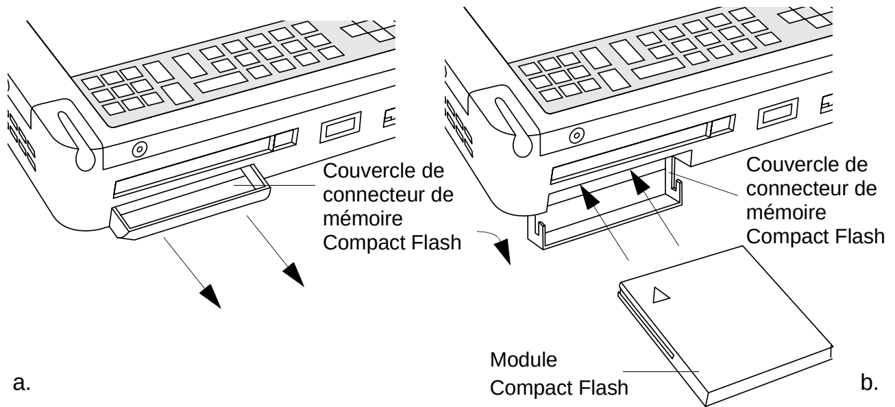
Figure 2-3 Installation d'un module de mémoire Compact Flash
