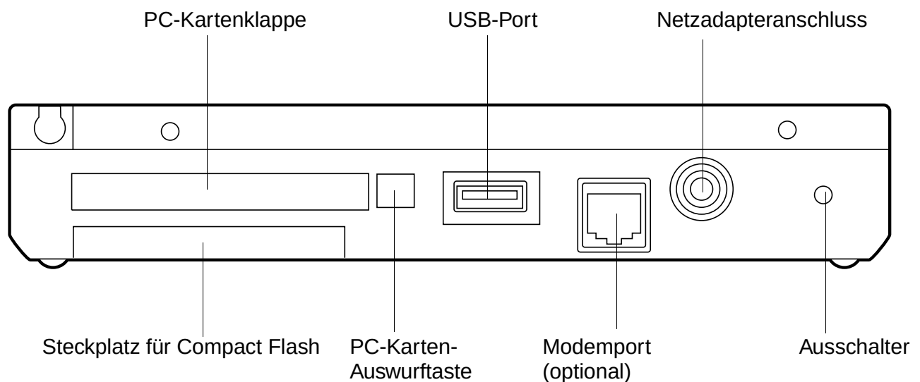
Abbildung 1-4 Anschlüsse und Schnittstellen auf der rechten Seite
