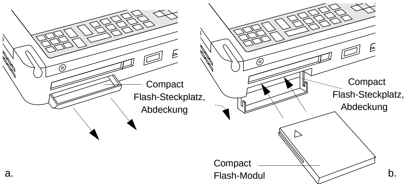
Abbildung 2-3 Installieren eines Compact Flash-Moduls
