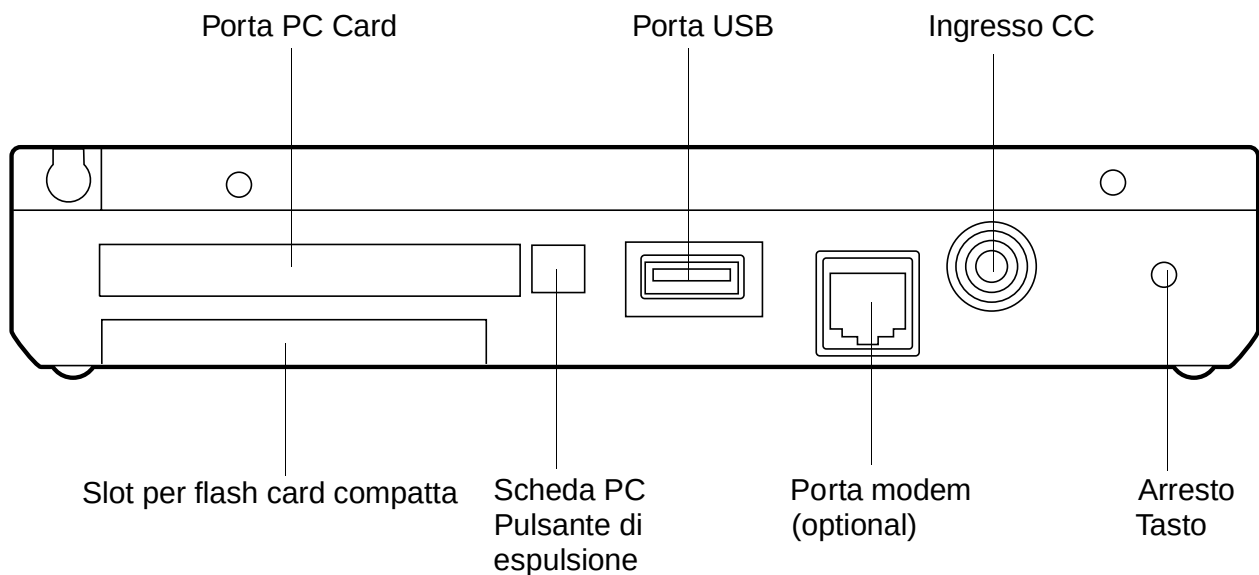
Figura 1-4 Connettori e interfacce lato destro
